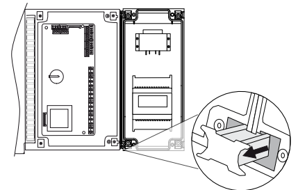
Beispiel mit UltraCella + Ultra-EVD-Modul
